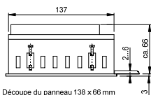
Découpe du panneau 138 x 66 mm
